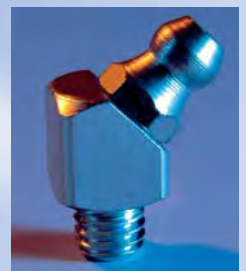
Kegelkopf-Schmiernippel nach DIN 71412
