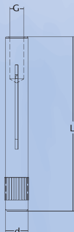
Schmierstifte mit Innengewinde, Rändel und Schmiernut Material S235JR
