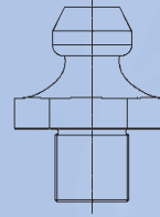
Kegelkopf-Schmiernippel, ähnlich DIN 71412
