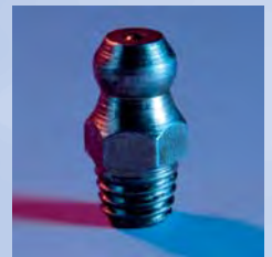
Kegelkopf-Schmiernippel, mit Selbstformgewinde nach DIN 71412
